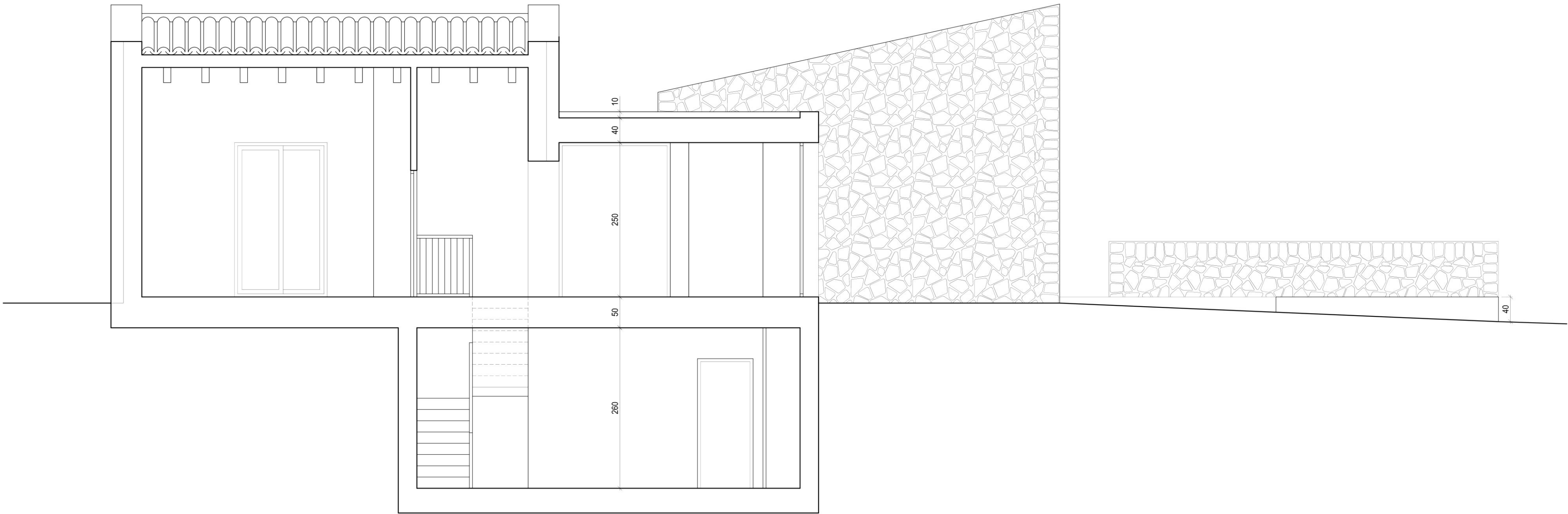
SECCION B-B'
