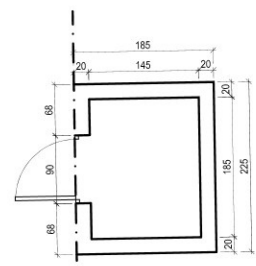
ESTACION TRANSFORMADORA SUP. CONSTRUIDA: 4,16 m 2
