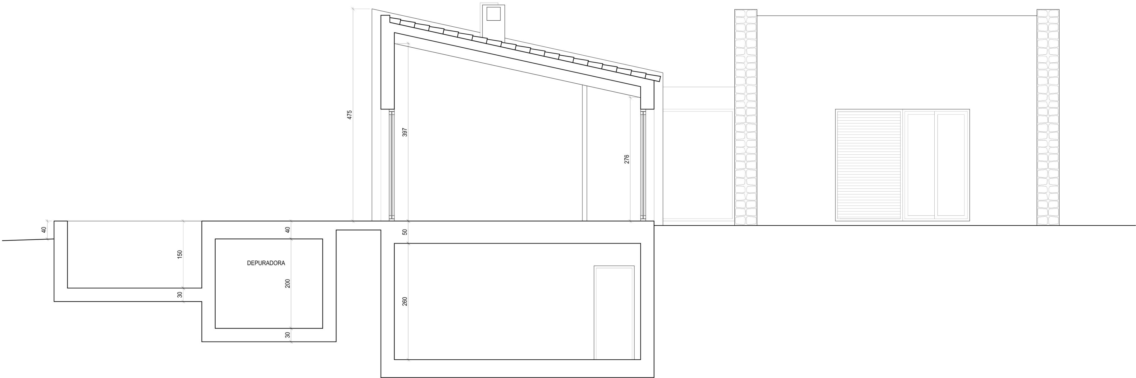
SECCION A-A'
