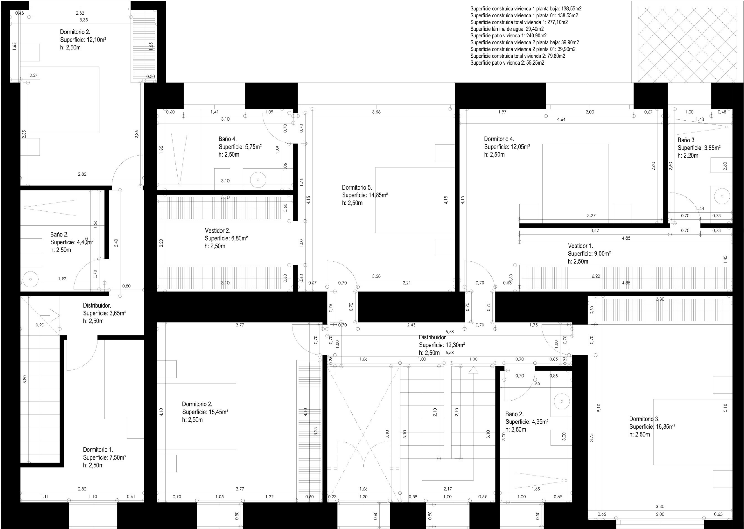
PLANTA 01. ESTADO PROPUESTO.
