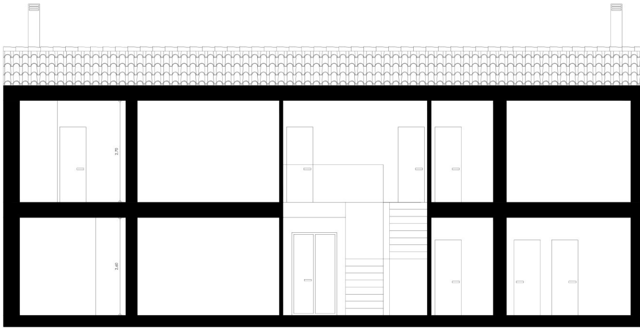
SECCIÓN A-A'. ESTADO PROPUESTO.
