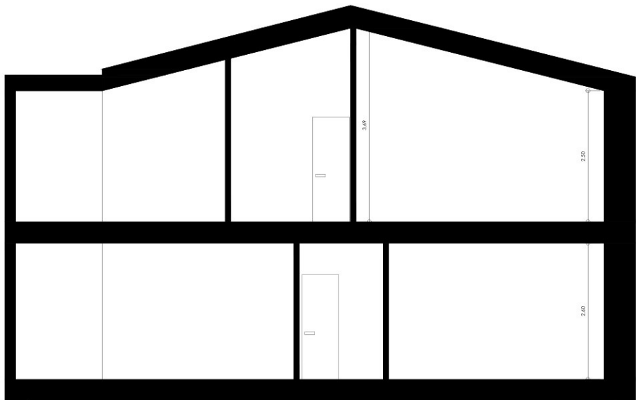
SECCIÓN C-C'. ESTADO PROPUESTO.
