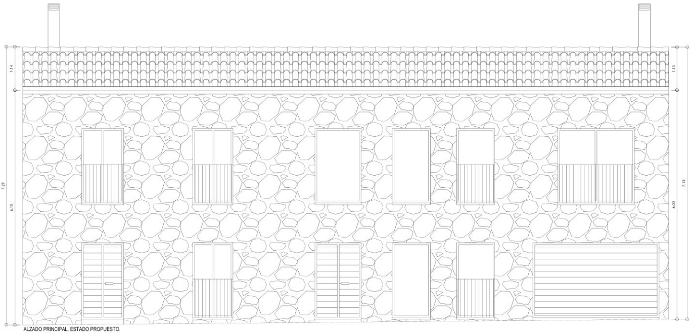
ALZADO PRINCIPAL. ESTADO PROPUESTO.
