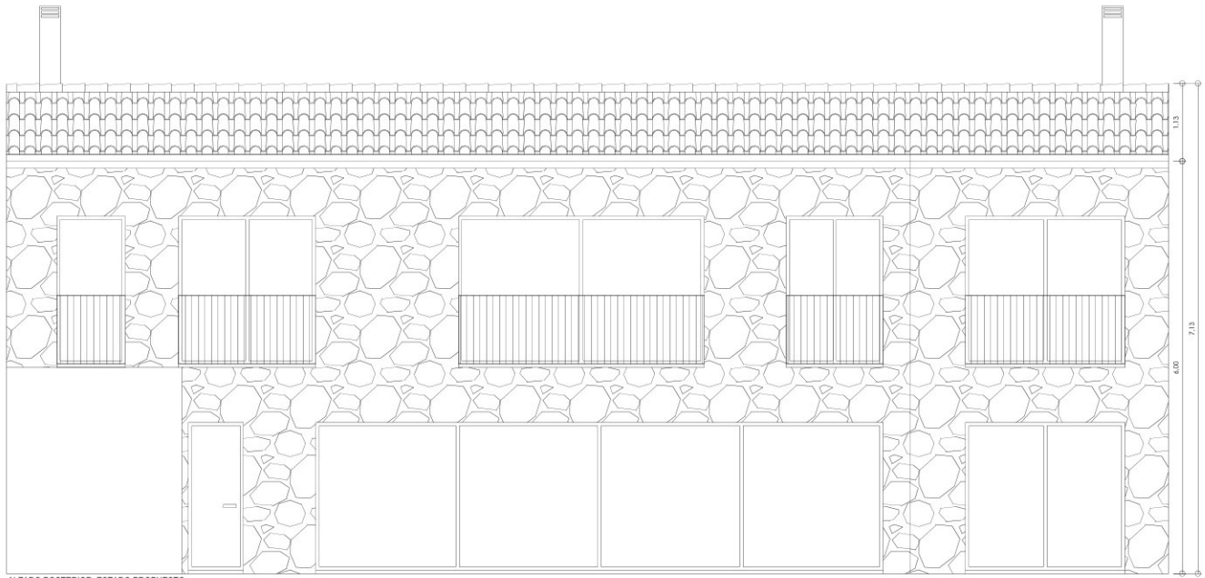
ALZADO POSTERIOR. ESTADO PROPUESTO.
